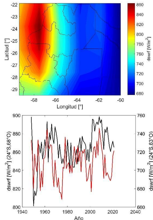
Figura 1. Promedio en el período 1948-2021 del promedio anual de dswrf (panel superior). Variación interanual del promedio anual de dswrf para dos puntos de la grilla: (24°S,68°O) (negro) y (24°S,63°O) (rojo).
